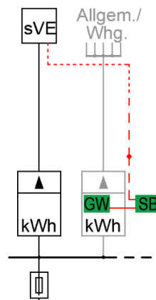
Bild 4: an Mehrkundenanlage oder EFH mit 2 Zählern
