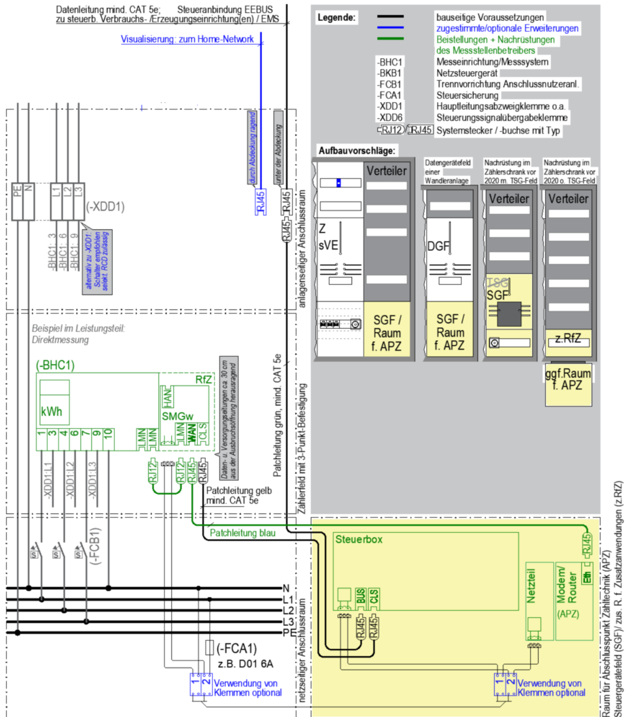
Abbildung 2: Anschlussplan (digitale Steuerung)
