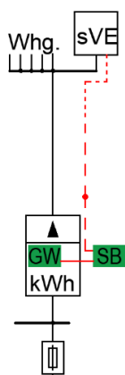
Bild 3: Gateway u. Steuerbox an Einkundenanlage
