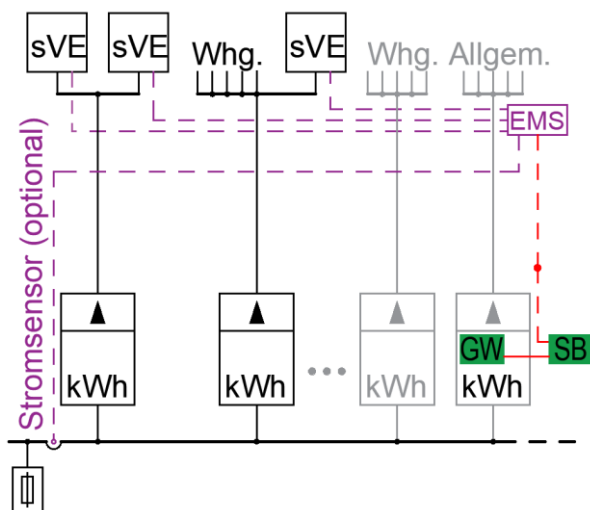
Bild 7: Prinzip Steuerung über EMS
