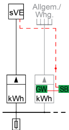
Bild 5: Prinzip direkte Steuerung für einzelne sVE
