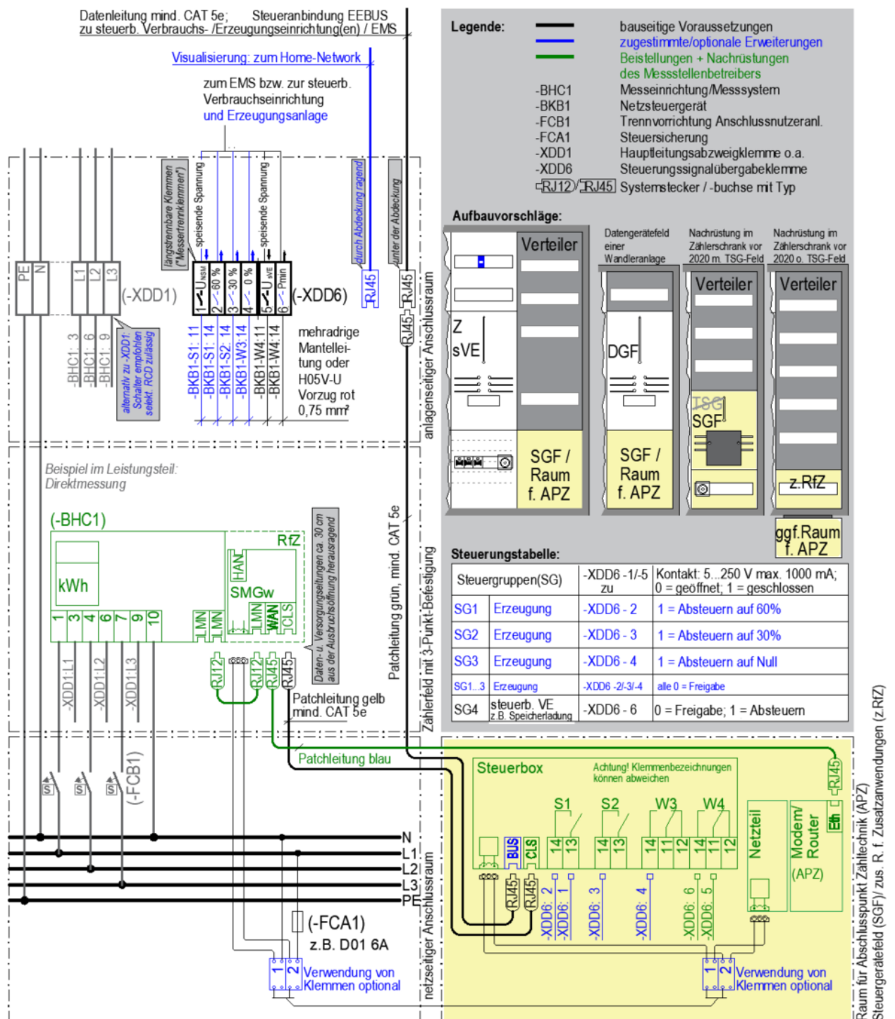
Abbildung 1: Anschlussplan (kontaktbasierte Steuerung)
