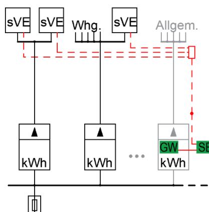
Bild 6: Prinzip direkte Steuerung als Gruppe
