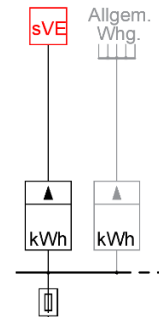
Bild 2: separater Zähler
